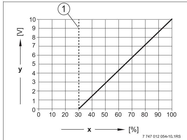
Рис. 17 Клемма U_{BR}
