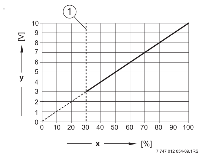
Рис. 14 Клемма U_{BR}
